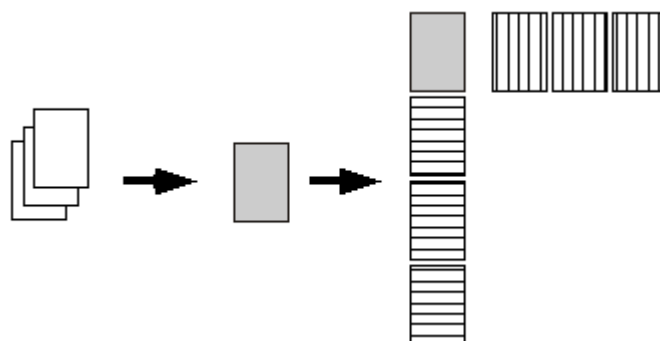
FIGURE 3 – En gris le tableau compromis dont l’analyse permet la projection en individus supplémentaires de toutes les lignes et la projection en variables supplémentaires de toutes les colonnes. On peut même projeter sur un plan des axes principaux du compromis les axes principaux de chaque tableau et sur le plan des composantes principales du compromis les composantes principales de chacun des tableaux.
