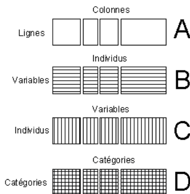
FIGURE 1 – K -Tableaux : un stockage commun pour des situations variées.
